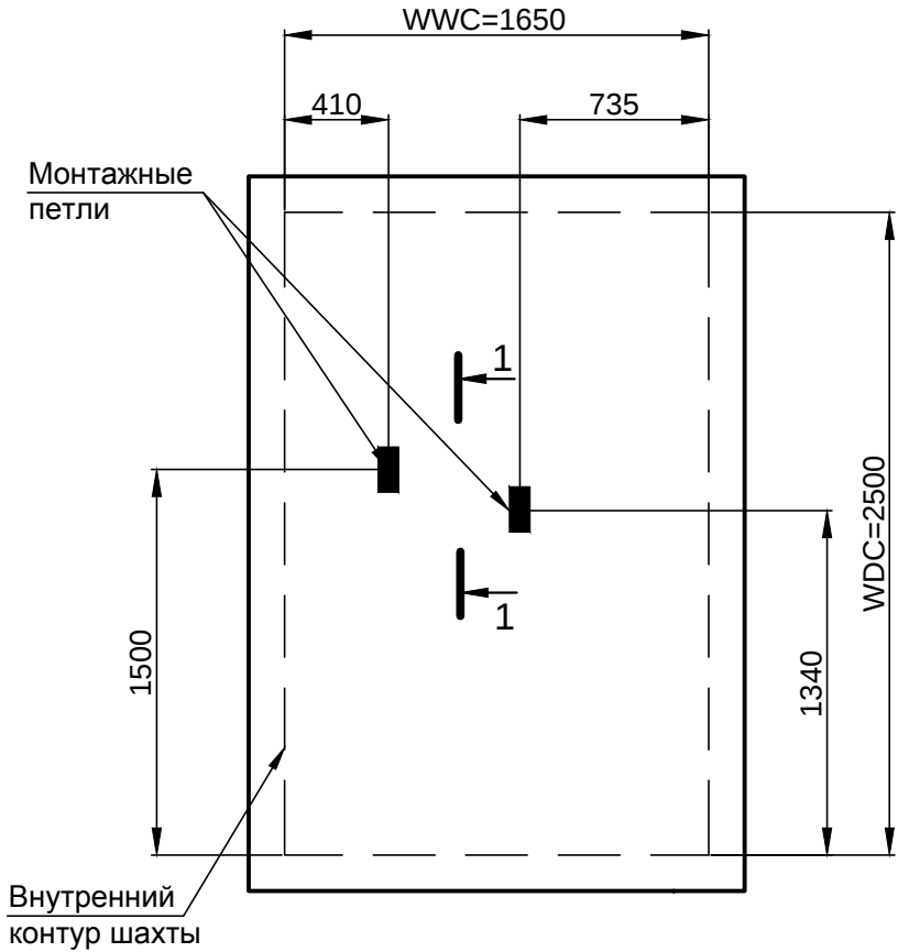
A - A (4) ○ (План расположения монтажных петель в перекрытии шахты)
