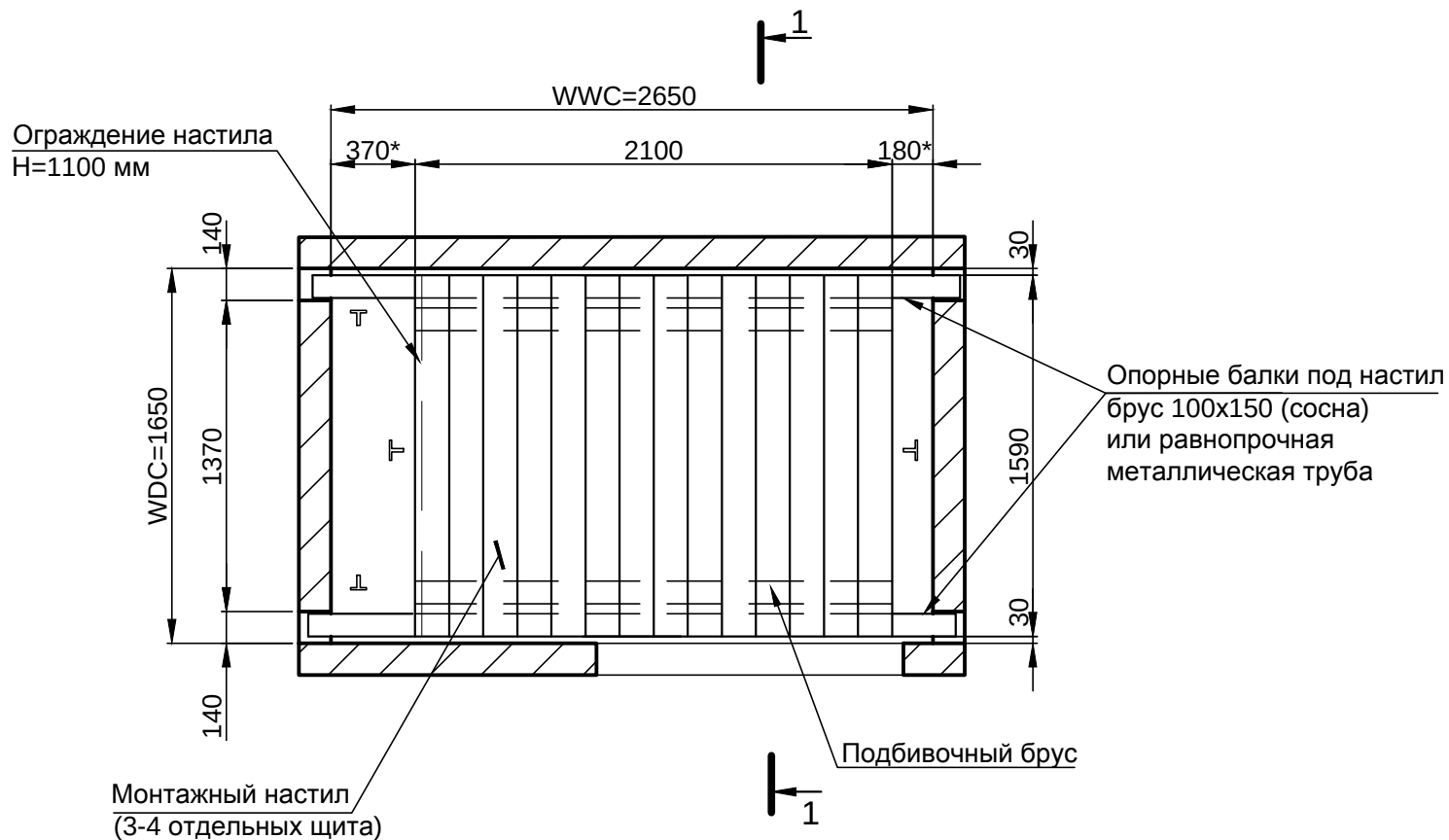
Схема расположения монтажного настила в шахте
