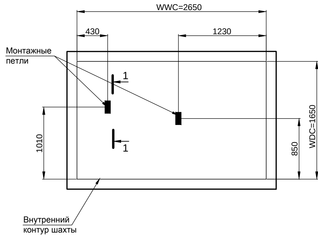
В - В (4) ○ (План приямка)
